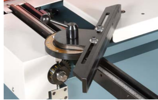
0-180° Açı Ayarlı Gönye
